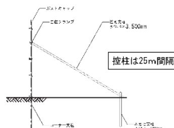
側面図 1/60
