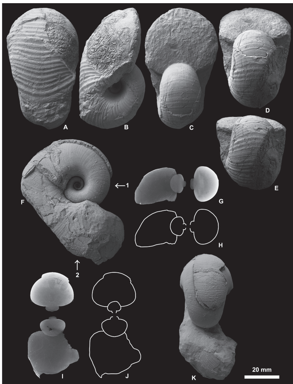
A-E, タカハシセラス第 4 標本 (HMG-2007)。F-K, タカハシセラス第 2 標本 (HMG-1524)。G, I は X 線 CT 画像。(研究報告第 36 号より転載)
