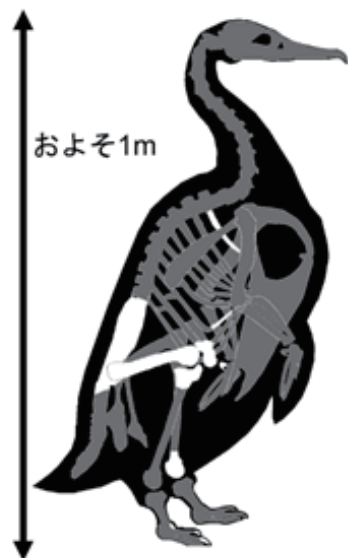
プロトプテルムの骨格図。 白抜きが産出した部位。
