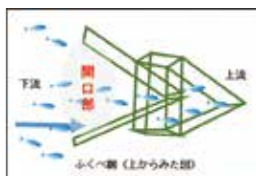
(図1) ふくべ網(左：鶴川に設置したふくべ網の写真 右：ふくべ網の図※矢印は川の流れを表しています)
