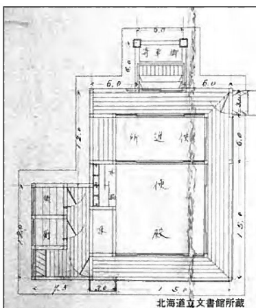
【図】鶴川昼餐休憩所平面図(北海道立文書館所蔵)
