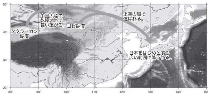
▲ 黄砂解説図
