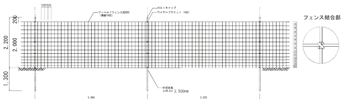
立面图 1/60
